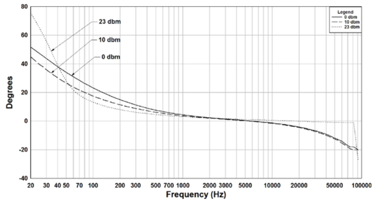
107N Rs=10K, RI=600 Phase Shift
