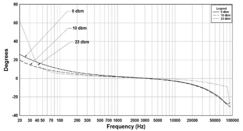
107P Rs=10K, RI=1500 Phase Shift
