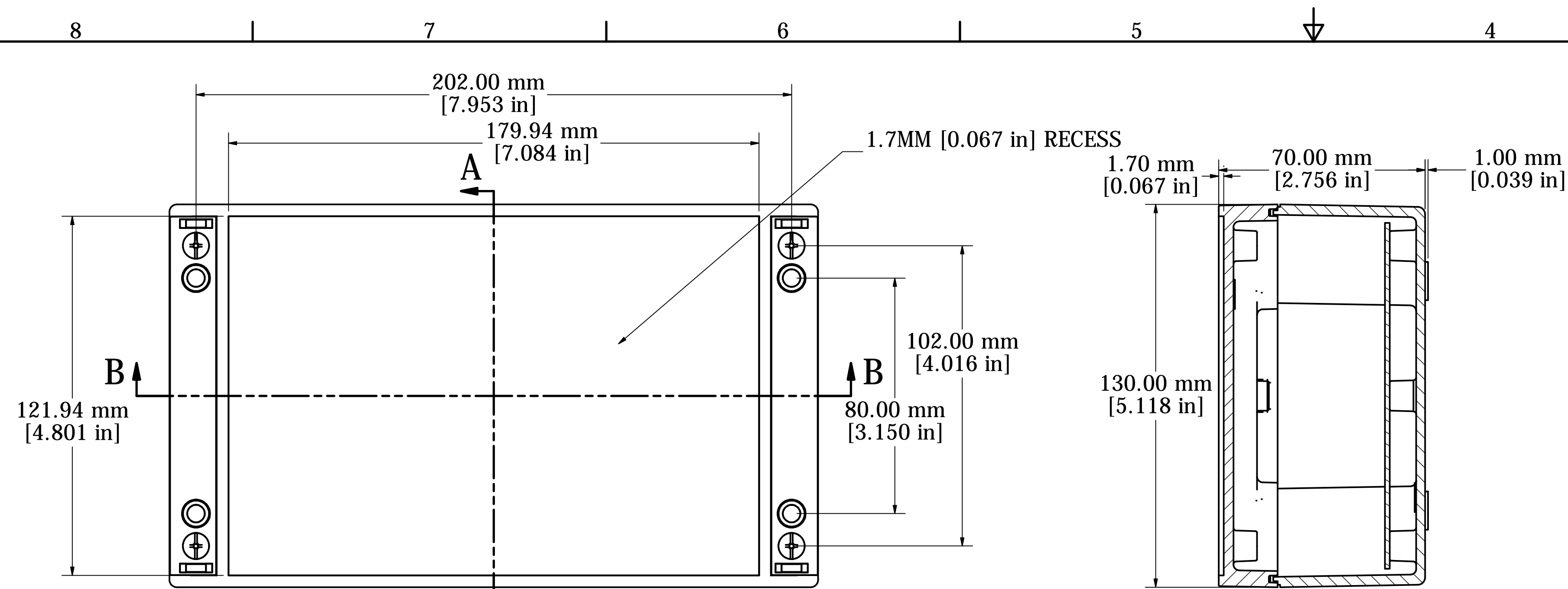
SECTION A-A
