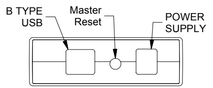
UNO/101 PANEL
